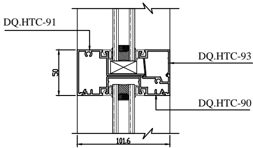
Section 2 Mặt cắt 2
