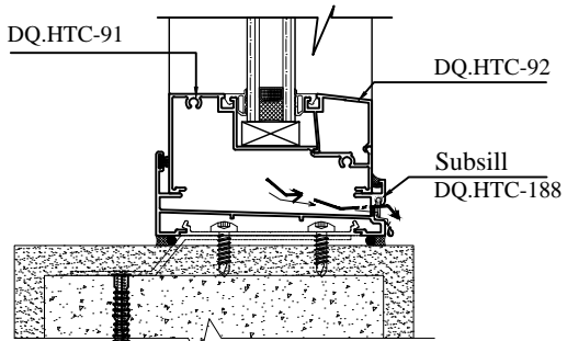
Section 3 Mặt cắt 3
