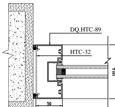
Section 4 Mặt cắt 4
