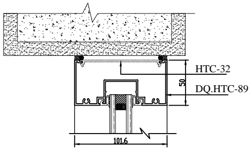
Section 1 Mặt cắt 1
