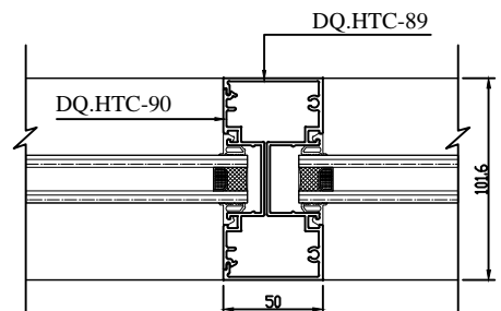
Section 5 Mặt cắt 5
